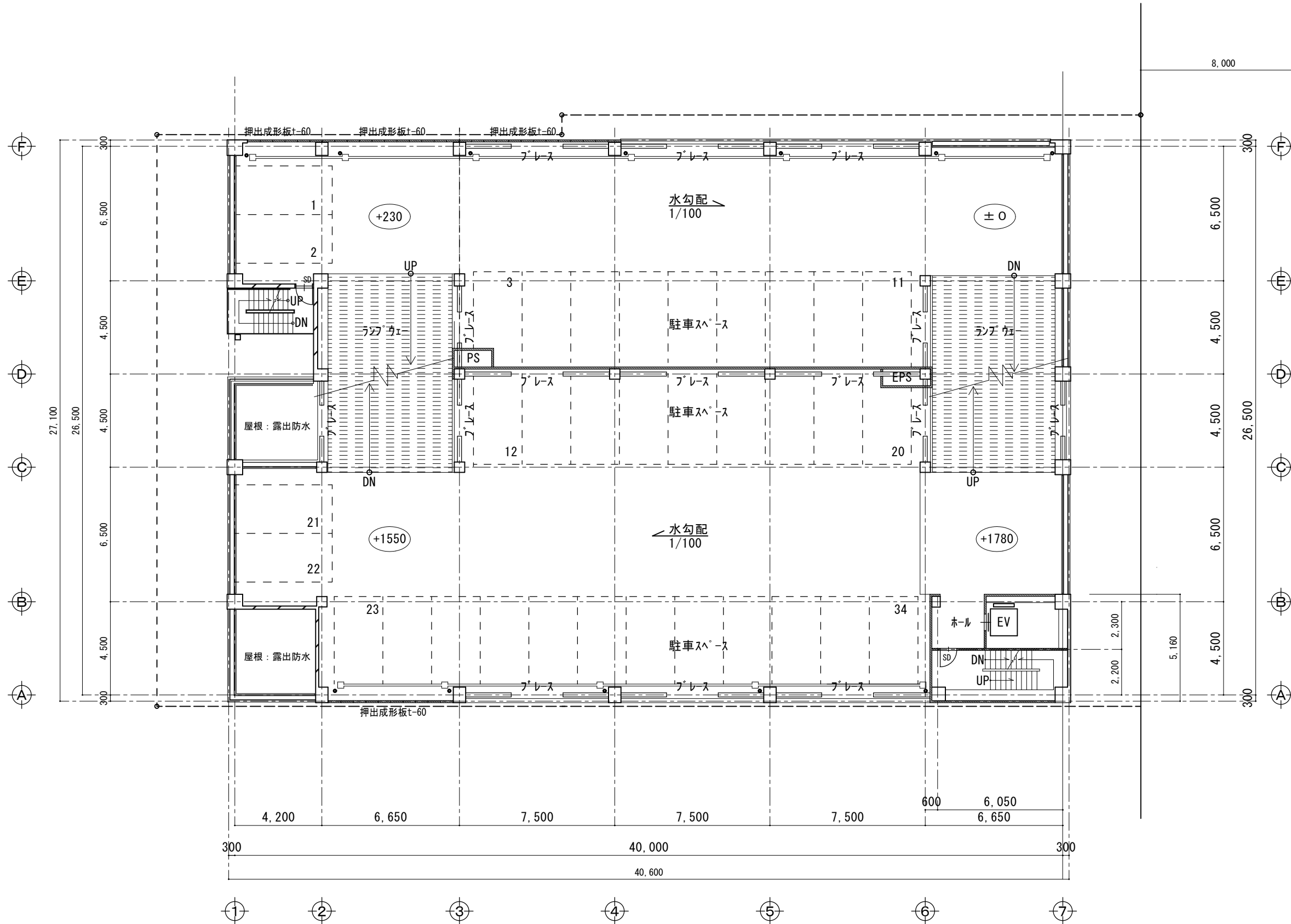
2 階 平 面 図 S=1/200 凡例 コンクリート壁厚150 押出成形板 t=60
