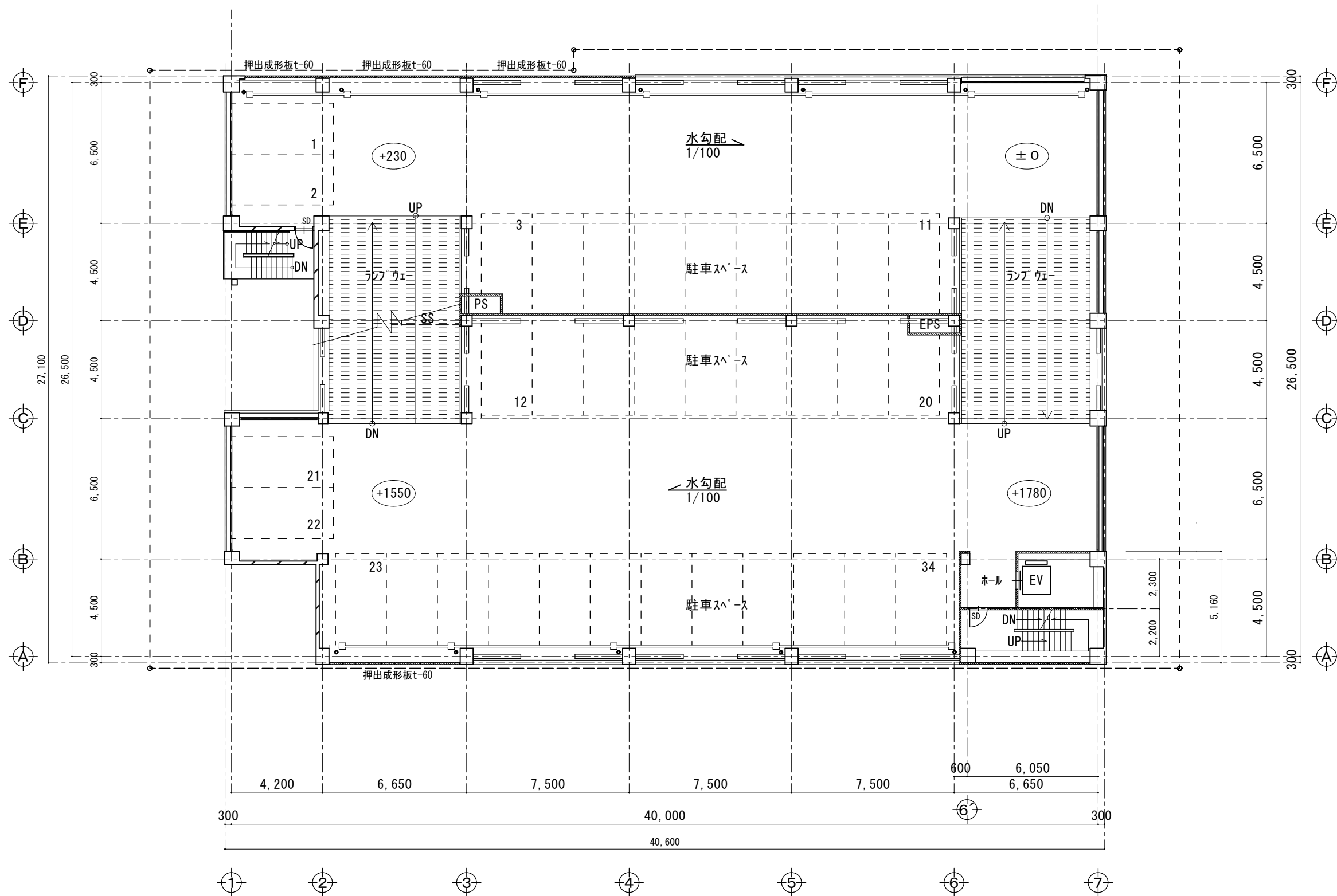
3 ~ 5 階 平 面 図 S=1/200 凡例 \rule{1cm}{0.4pt} → コンクリート壁厚 150 \rule{1cm}{0.8pt} → 押出成形板 t=60
