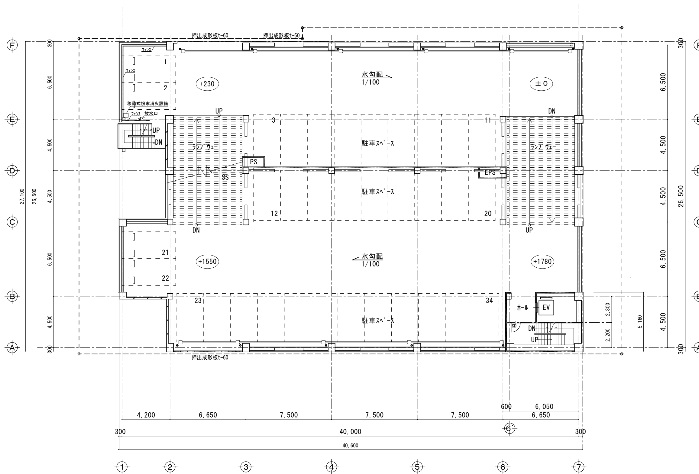
6 階 平 面 図 S=1/200 凡例 ——→ コンクリート壁厚150 ——→ 押出成形板t-60
