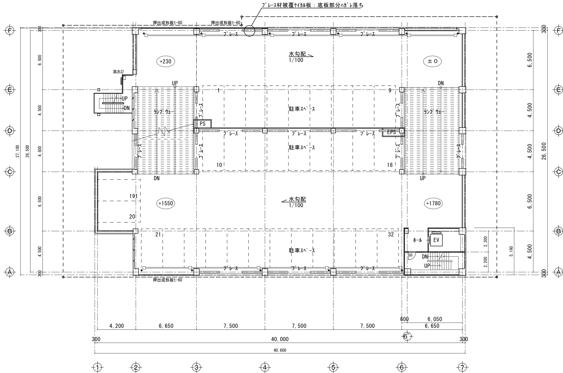
7 階 平 面 図 S=1/200 凡例 → コンクリート壁厚150 → 押出成形板t-60
