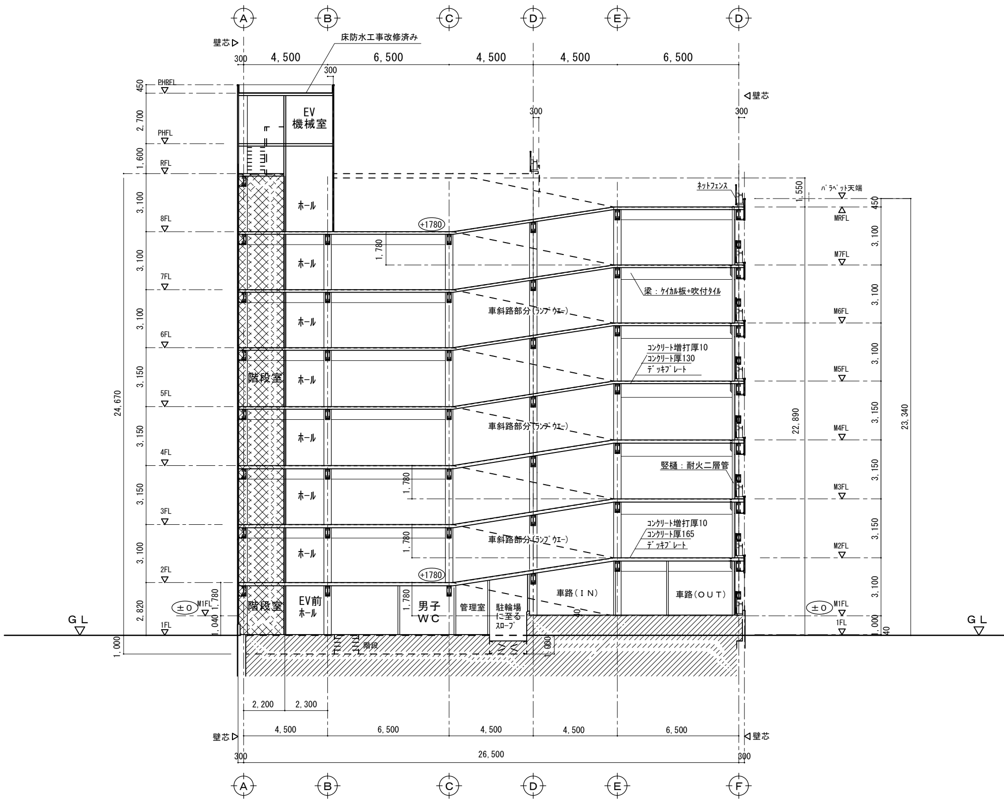
c-c 断面図 【6~7通り間】 S=1:200
