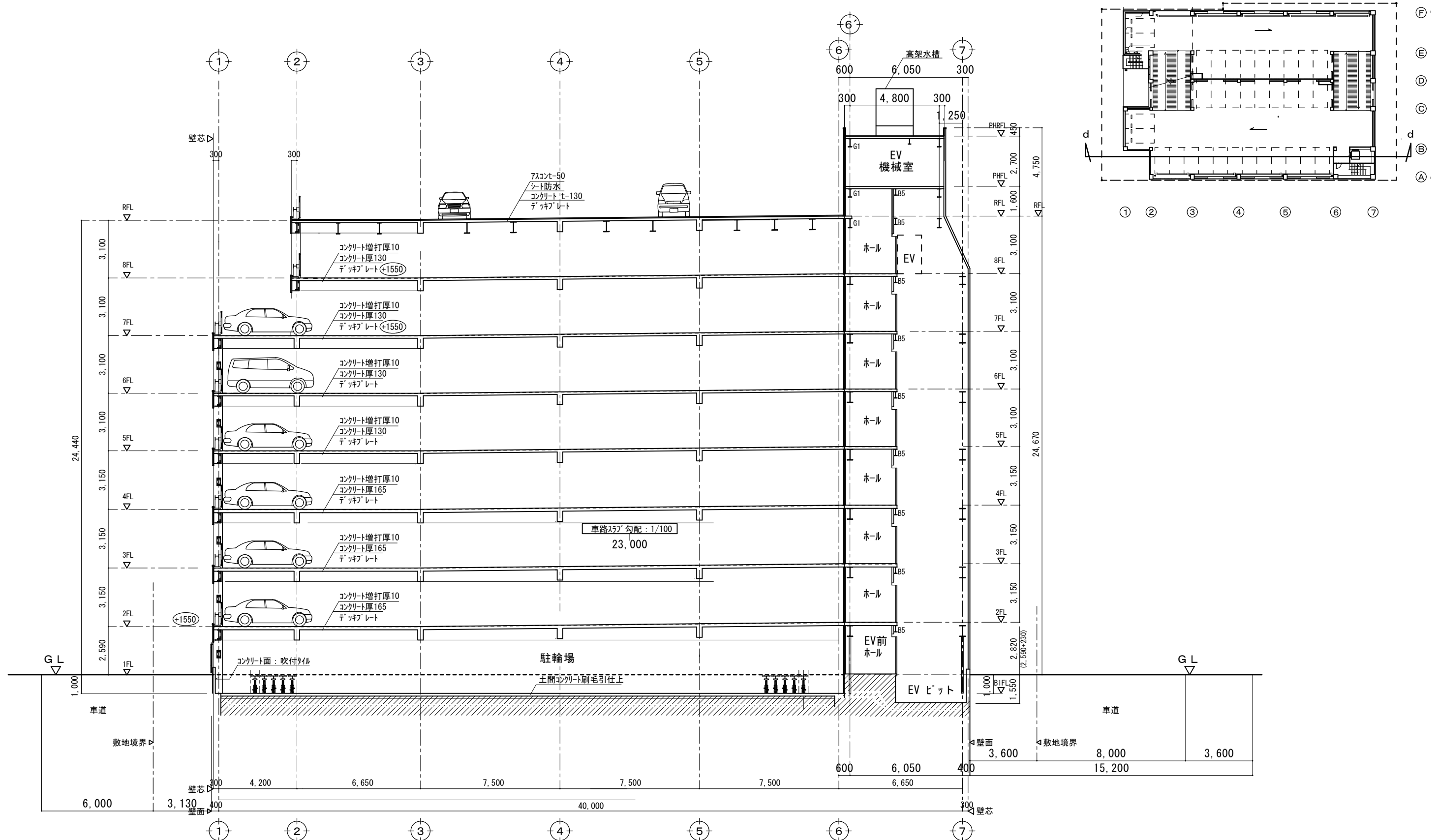
d-d 断面図 【A~B通り間】 S=1:200
