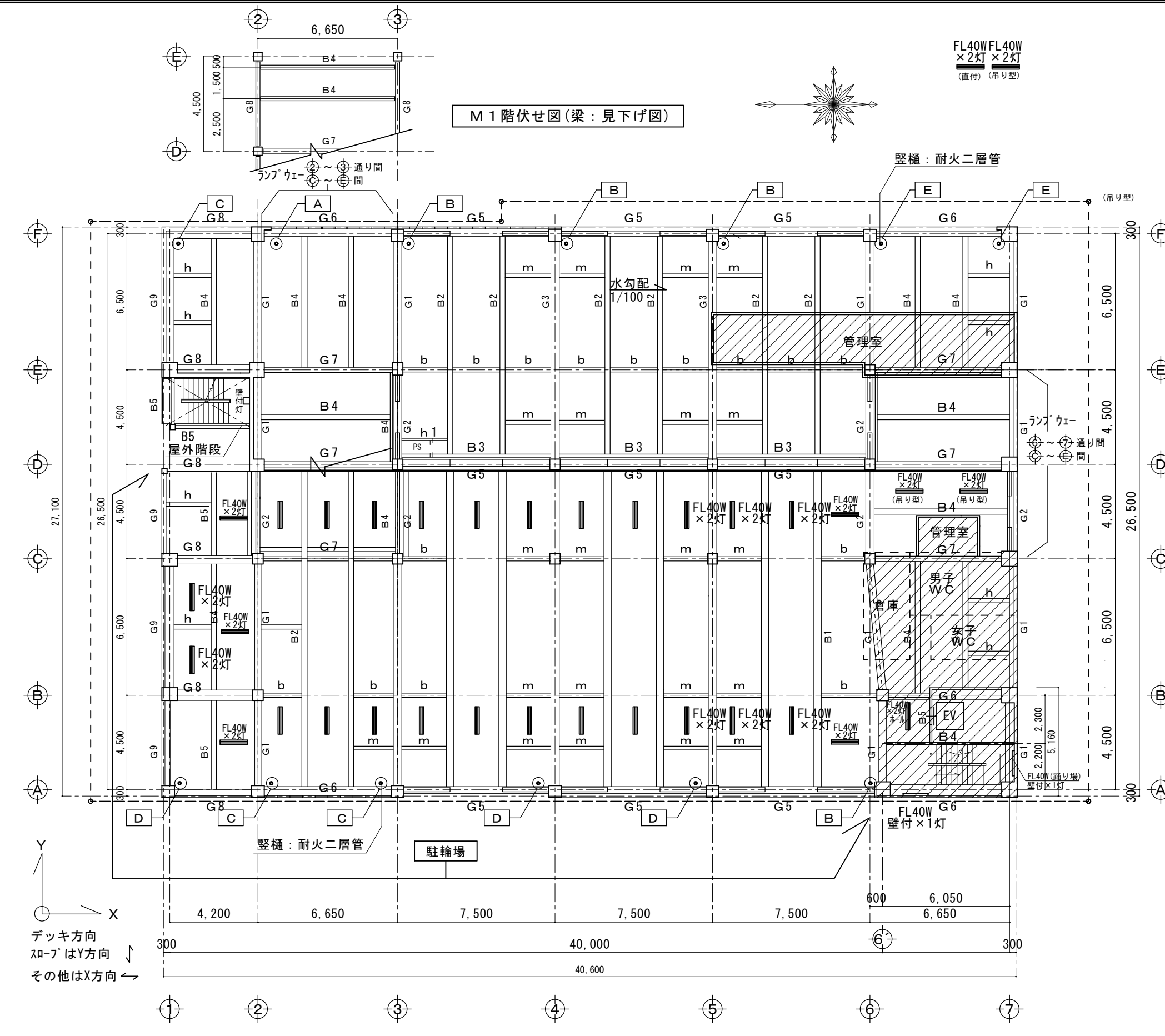
1階(2階床)梁伏図 S=1/200 (梁:見上げ図)
