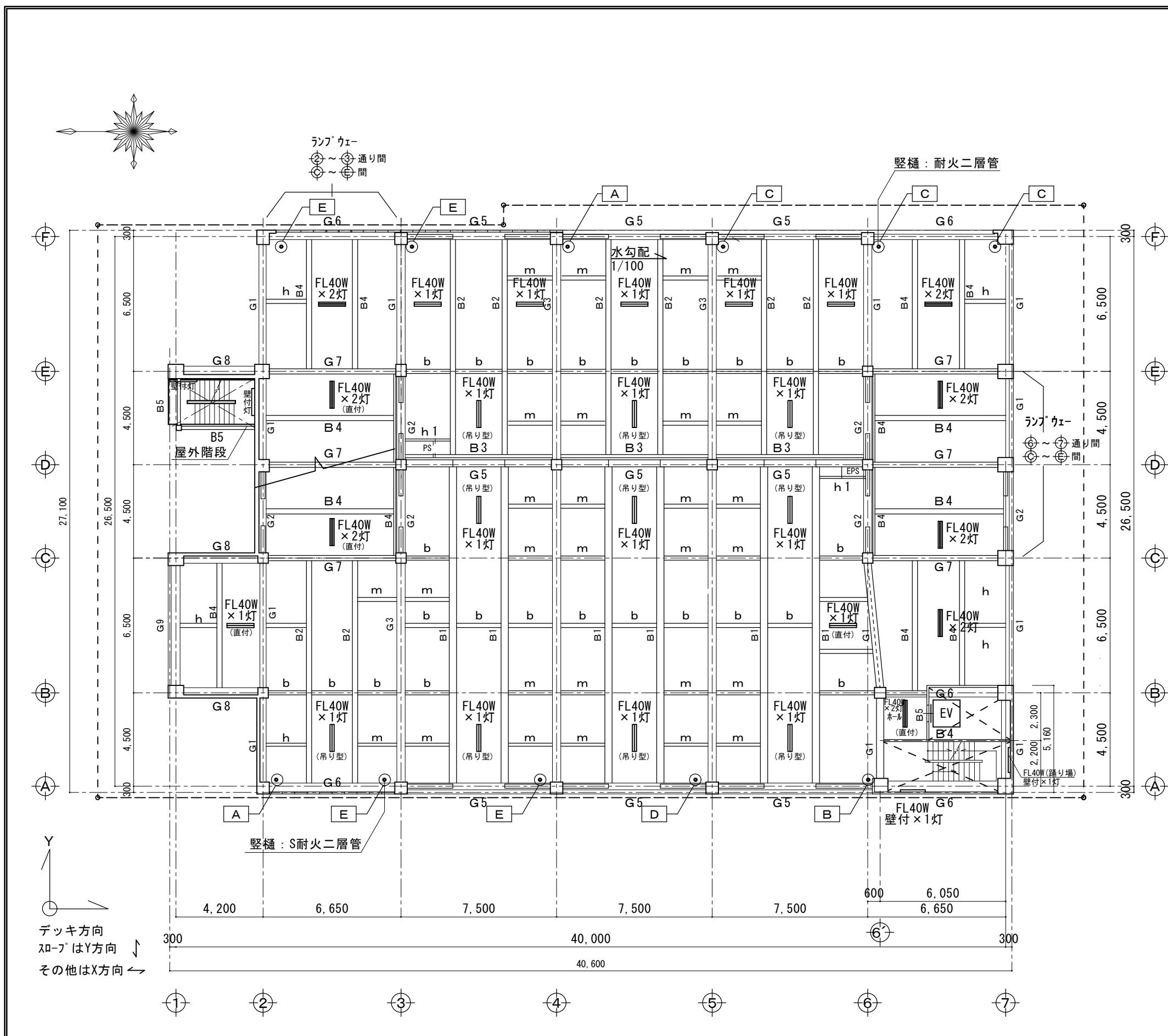
5階(6階床)梁伏図 S=1/200 (梁: 見上げ図)
